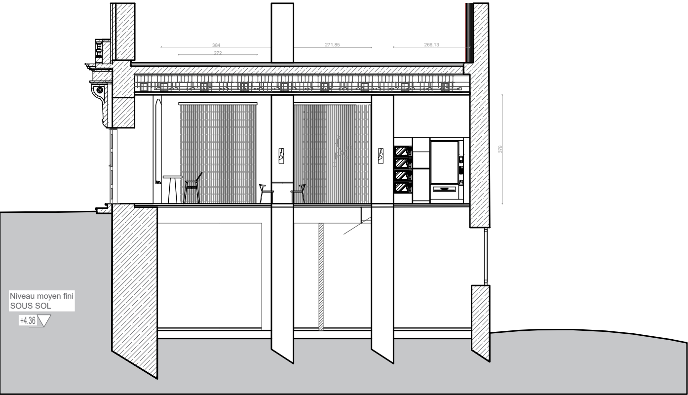
Coupe CC
