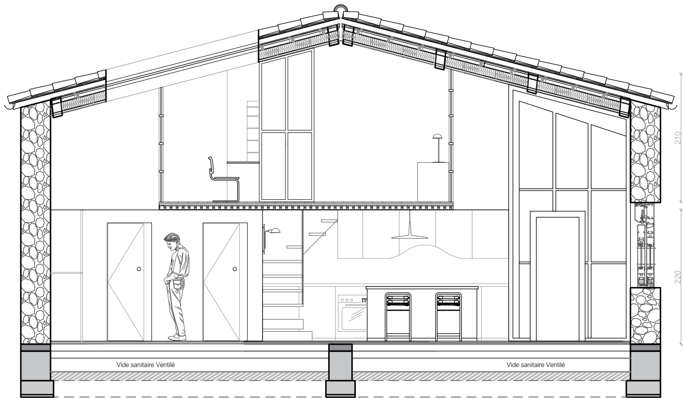
Coupe AA
