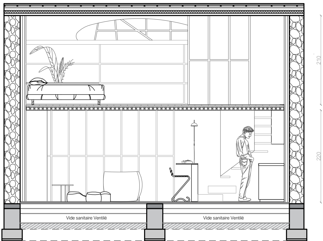
Coupe BB
