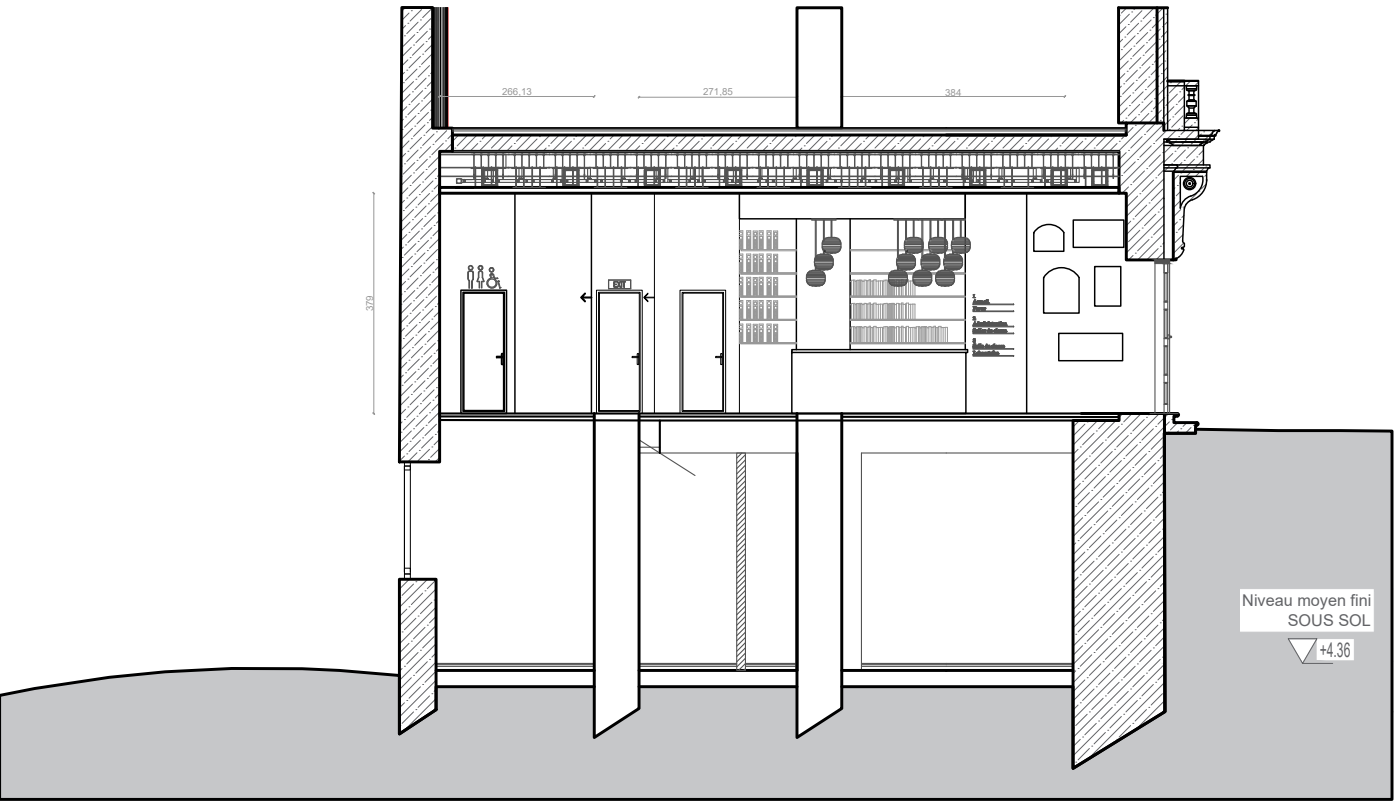
Coupe DD
