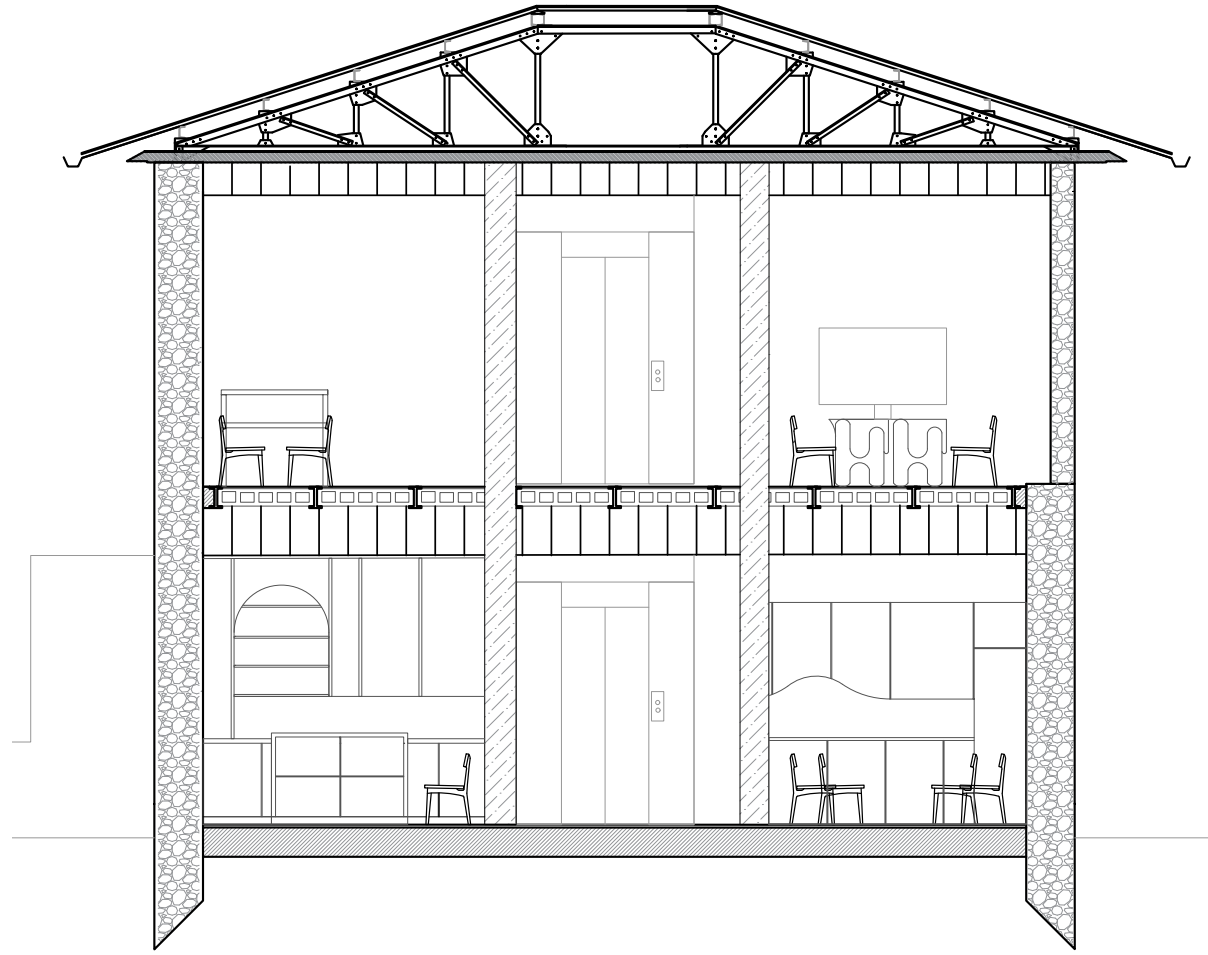
Coupe AA
